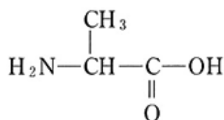
アラニン
