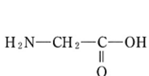
グリシン
